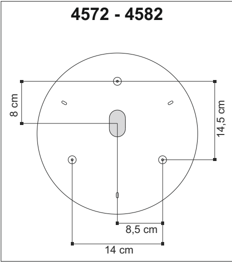
Schema per il fissaggio per installazione singola Mounting layout for single installation
