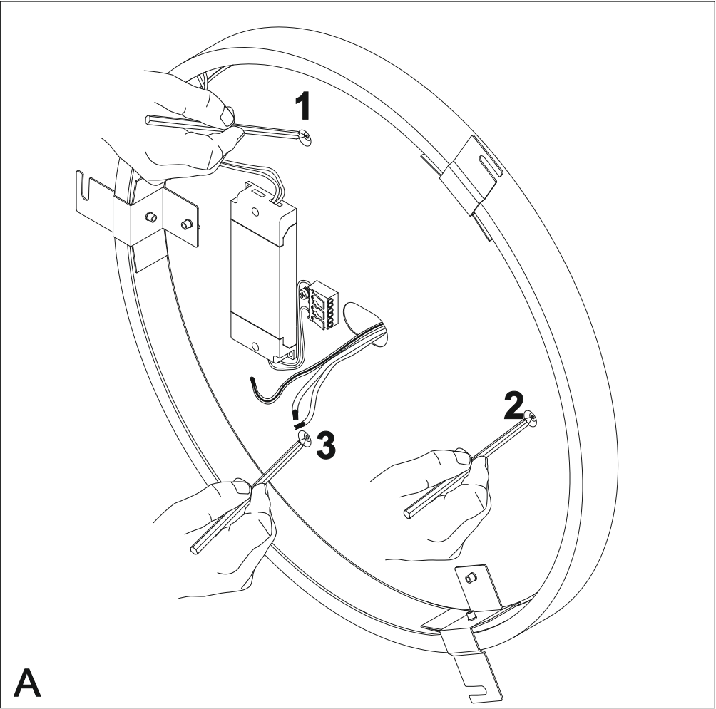
Schema per il fissaggio per installazione singola Mounting layout for single installation
