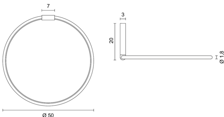
Dimensioni - Dimensions
