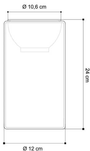
Dimensioni del diffusore - Diffuser dimensions
