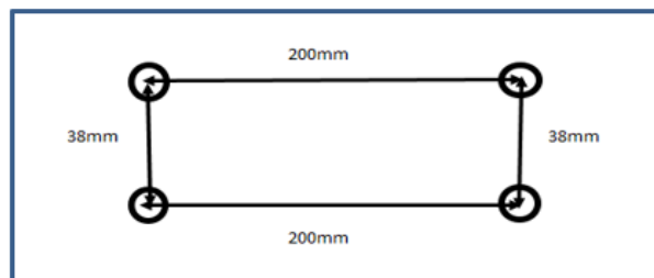
Befestigungslöcher, Fixing holes 160-007-70/160-007-40
