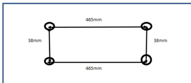
Befestigungslöcher, Fixing holes 160-008-70 / 160-008-40
