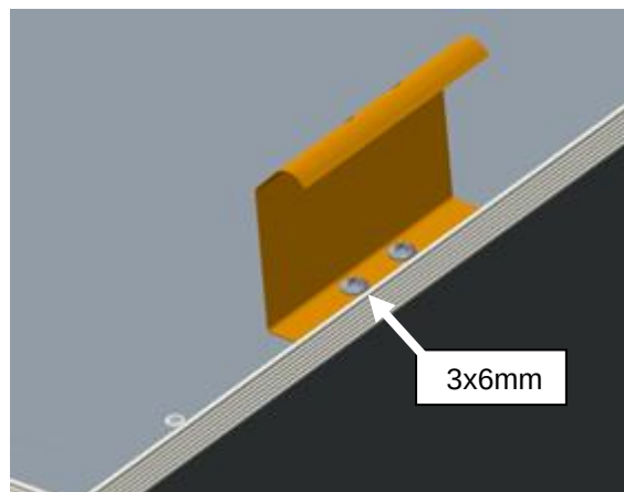
160-013-96 Gema-Armstrong Q-Clip
